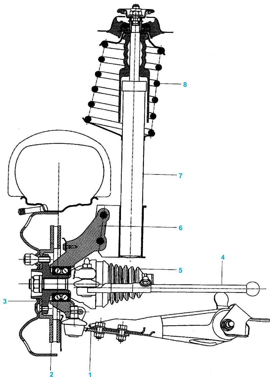
1 : Bras inférieur - 2 : Disque de frein - 3 : Moyeu de roue - 4 : Bielle de direction - 5 : Demi-arbre de transmission - 6 : Porte-fusée - 7 : Amortisseur - 8 : Ressort hélicoïdal de suspension
