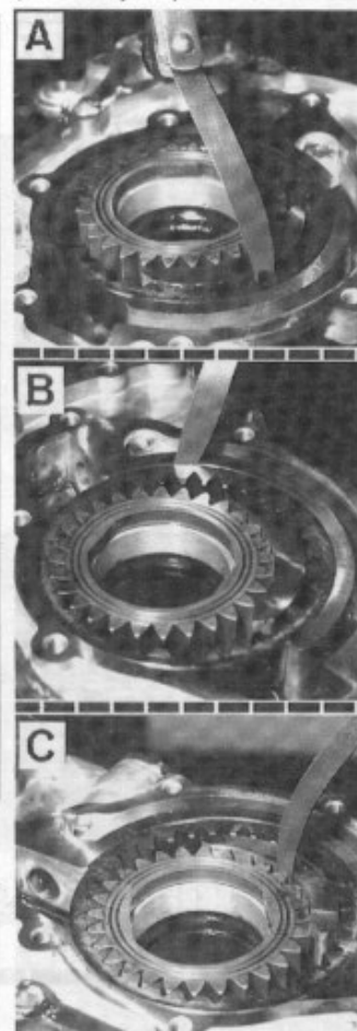
Contrôle du jeu radial A et B. Entre pignon extérieur et carter - C. Entre pignon intérieur et carter.
