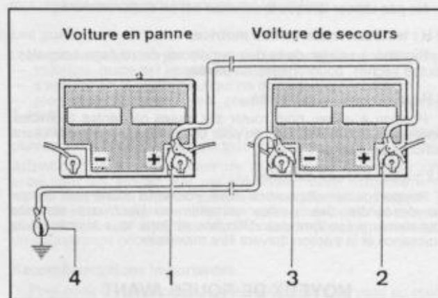
Démarrage du moteur à l'aide d'une batterie auxiliaire A. Batterie déchargée - B. Batterie de secours - 1, 2, 3, 4, ordre de branchement (le 4 correspond à une pièce métallique du moteur du véhicule défaillant).
