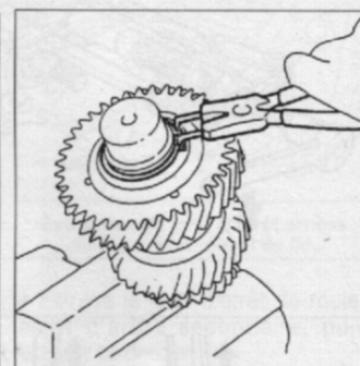
Dépose du jonc d'arrêt de l'arbre secondaire.
