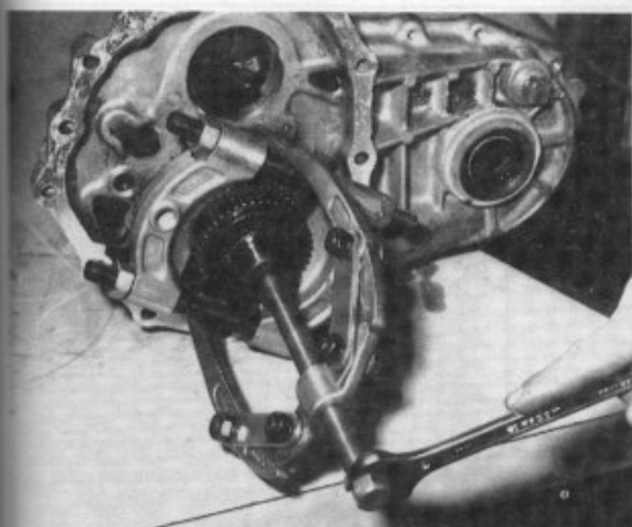
Extraction du moyeu de rapport long/court.
