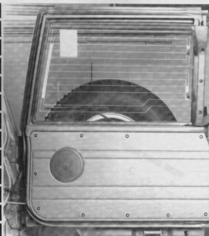
Points de fixation des garnitures de portes arrière
