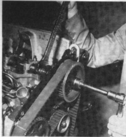
Immobilisation de l'arbre à cames et dépose du pignon.
