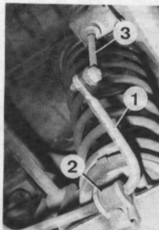
Dépose de la barre stabilisatrice 1. Barre stabilisatrice - 2. Pailier - 3. Biellette.
