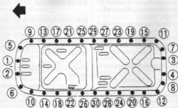
Dépose du carter d'huile : Ordre de desserrage Flèche : Côté distribution.
