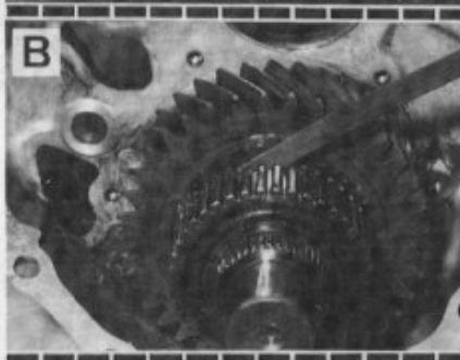
Choix d'un segment d'arrêt d'arbre primaire.
