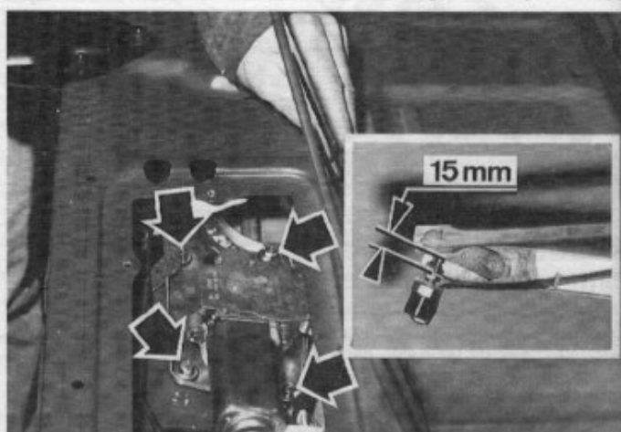
Fixations du mécanisme d'essuie-glace arrière et réglage de l'interrupteur de rappel (Patrol 260).
