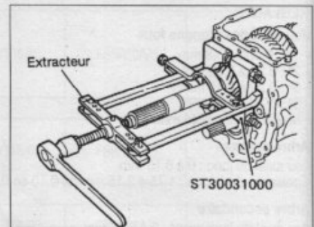
Extraction du pignon de 5 e .
