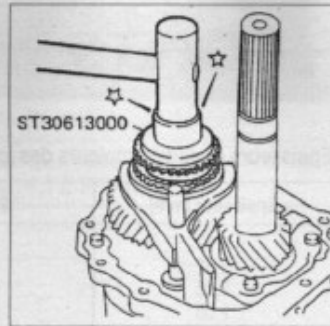
Repose du cône et de la rondelle de synchronisation de 5 e .
