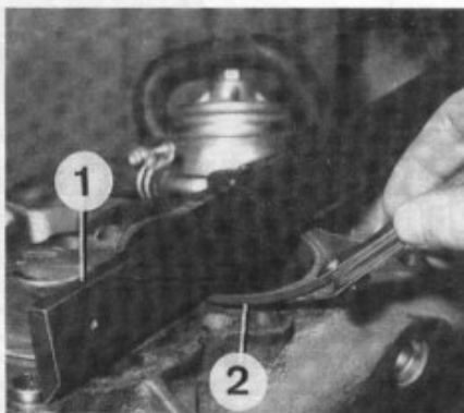
Contrôle de la planéité du bloc-cylindres 1. Règle - 2. Jauge d'épaisseur.
