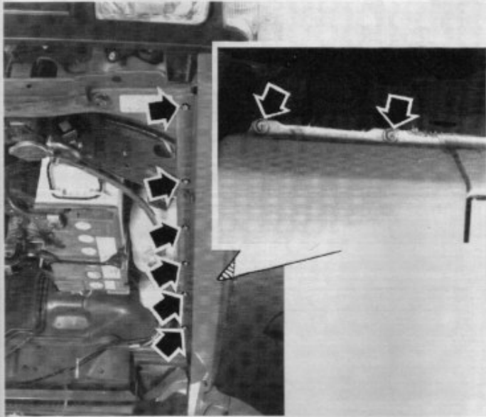
Fixations d'une aile avant de Patrol 260. Deux vis de fixation sous le bouclier ne sont pas repérées
