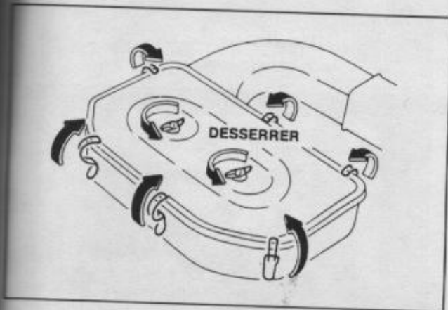
Remplacement de la cartouche filtrante du filtre à air (Photo RTA) Ci-dessus : sur 260 - Ci-dessous : sur GR.
