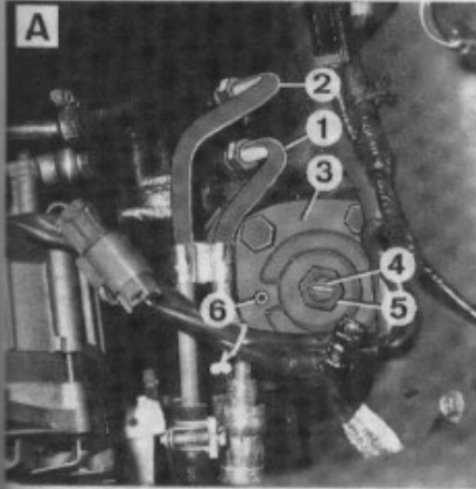
Boîtier de direction en place sur véhicule A. Patrol 260 - B. Patrol GR.
