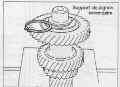
Choix d'un jonc d'arrêt pour minimiser le jeu d'arbre intermédiaire.
