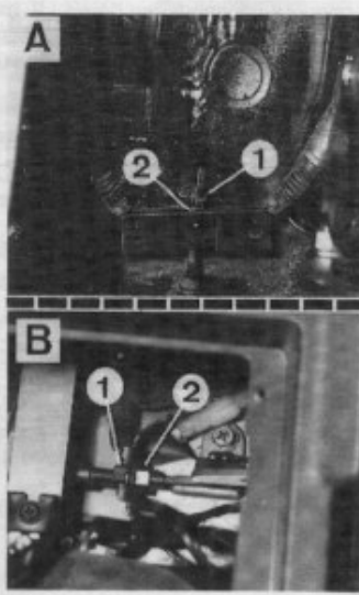
Réglage du frein de stationnement A. Patrol 260 - B. Patrol GR. 1. Contre-écrou - 2. Ecrou de réglage.
