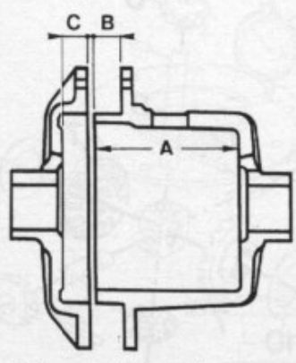
Cotes caractéristiques des carters (pont H 233 B).
