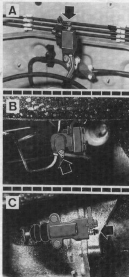
Purge de la commande hydraulique A. Purge supérieure (Patrol GR) - B. Amortisseur de pulsation (Patrol 260) - C. Cylindre récepteur.
