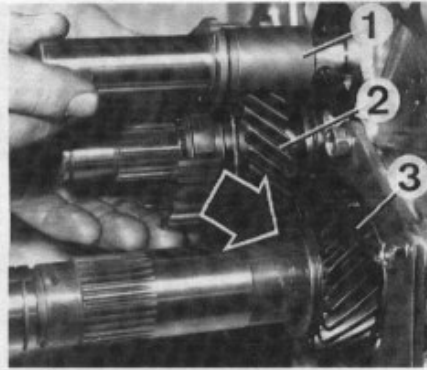
Montage du pignon de 5° - (3) orienter le grand collet (flèche) vers l'arrière - Montage simultané de l'axe du pignon de renvoi de M.A.R. - (1) et du pignon fou de 5° (2).
