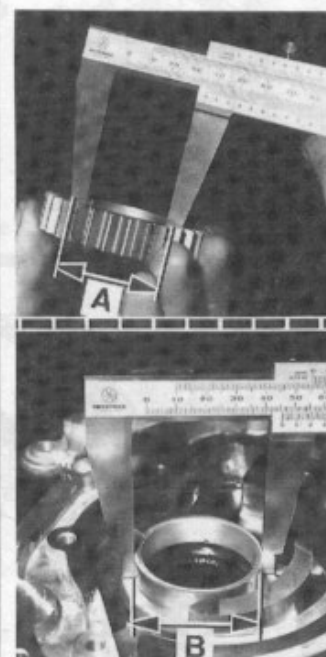
Contrôle du jeu radial du pignon intérieur Jeu = A-B.
