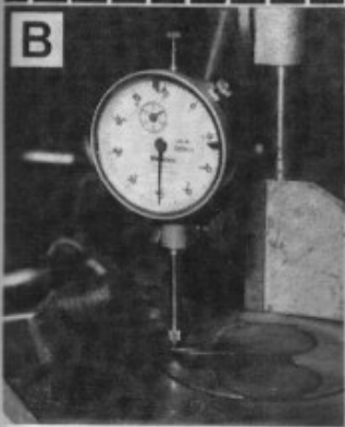
Contrôle du dépassement des pistons.
