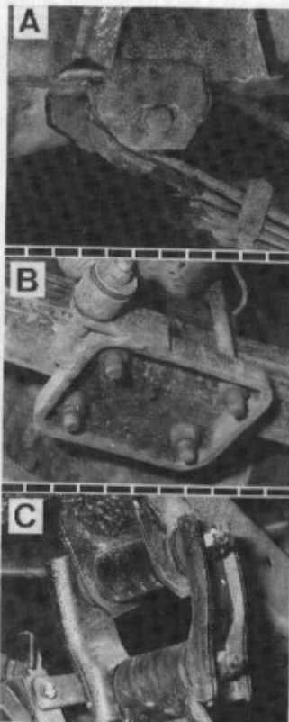
Fixations d'un ressort à lames A. Fixation avant - B. Fixation sur le pont - C. Fixation arrière.
