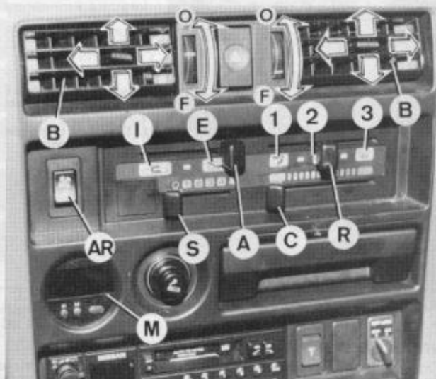
Commandes d'aération - chauffage sur GR (Photo RTA)
