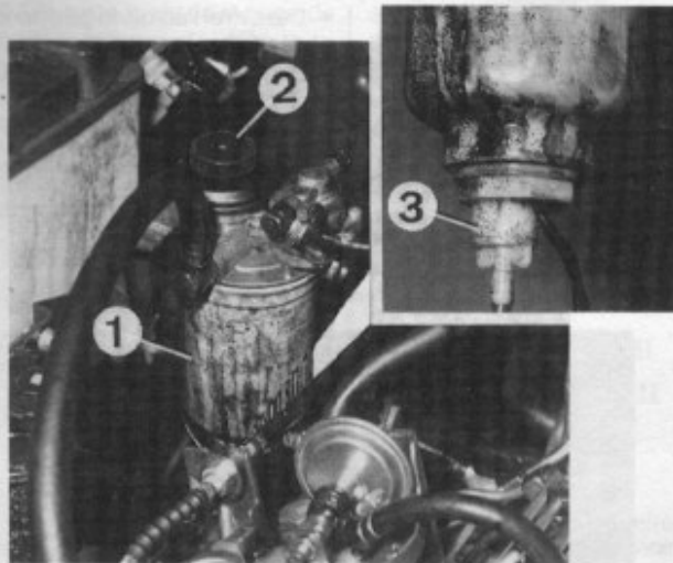
Purge du circuit de combustible 1. Filtre - 2. Pompe d'amorçage - 3. Robinet de purge de l'eau.
