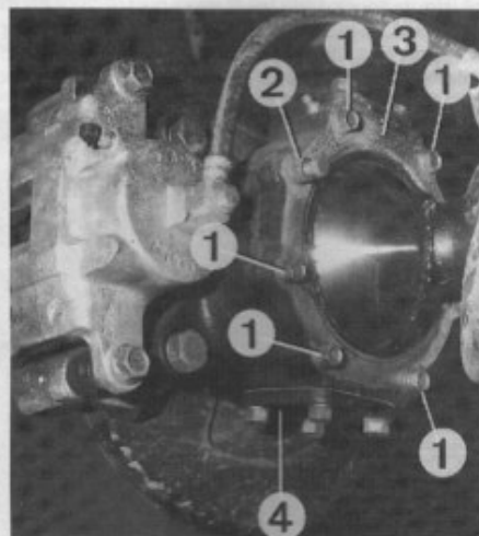
Montage du pivot 1. Vis de fixation des demi-flasques - 2. Vis de butée de braquage maxi - 3. Demi-flasques d'étanchéité - 4. Couverture de roulement de pivot.
