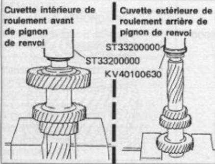
Repose des roulements avant et arrière d'arbre intermédiaire.
