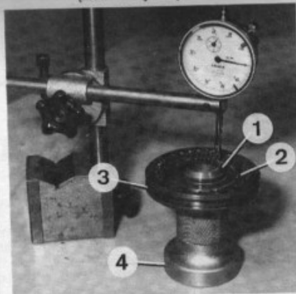
Contrôle de l'usure de la bague de synchro de M.A.R.
