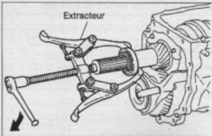
Extraction du roulement arrière d'arbre secondaire.
