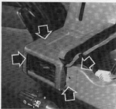
Implantation des agrafes de maintien du revêtement supérieur de planche de bord.
