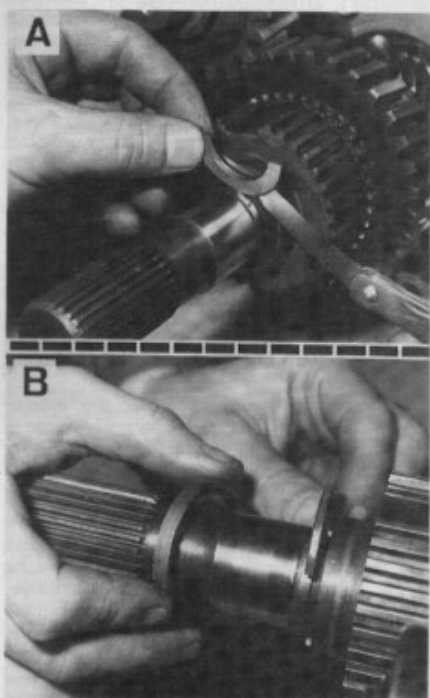
Montage des demi-anneaux d'arrêt A. Mesure du jeu et choix des demi-anneaux - B. Montage des demi-anneaux.
