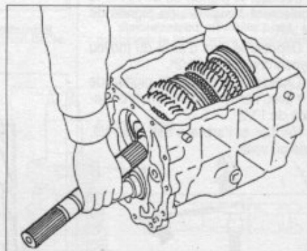
Dépose de l'ensemble arbre secondaire.
