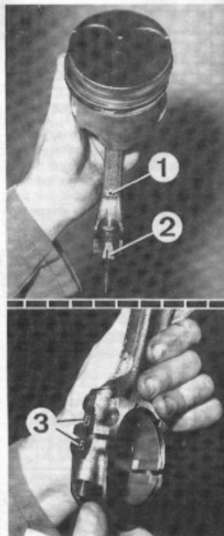
Repérage bielle-piston 1. Gicleur d'huile - 2. Repère d'alésage des têtes de bielle - 3. Repère d'identification des cylindres.
