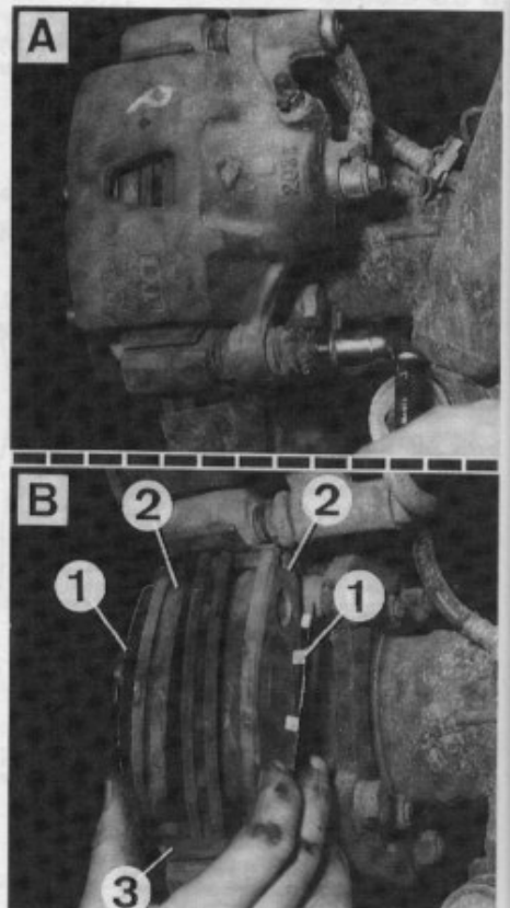
Remplacement des plaquettes de freins A. Dépose de la vis de colonnette inférieure - B. Dépose des plaquettes. 1. Plaque anti-bruit - 2. Plaquettes - 3. Ressort de retenue.
