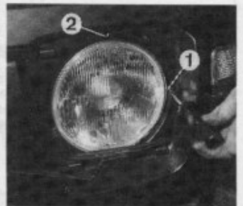
Réglage des projecteurs (disposition des vis identiques sur Patrol GR et Patrol 260) 1. Vis de réglage horizontal - 2. Vis de réglage vertical.
