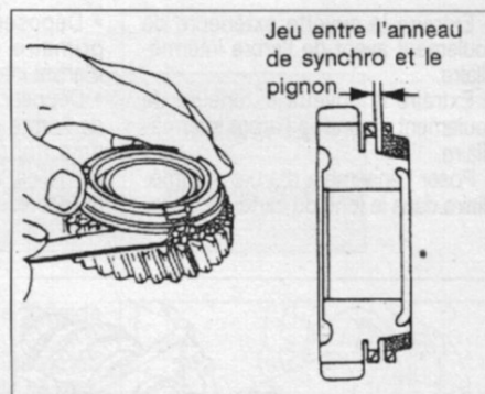
Mesure du jeu entre les bagues de synchronisation et les pignons (1 re , 2 e , 3 e et M. AR).
