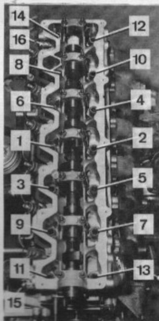
Ordre de serrage des vis de culasse.
