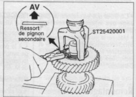
Repose de la rondelle élastique (face concave côté couronne dentée) avec le jonc d'arrêt choisi.
