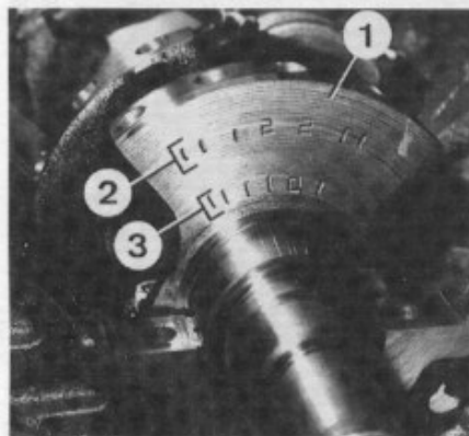
Repère d'image du vilebrequin 1. Masse d'équilibrage du cylindre n° 6 - 2. Repère des classes des manetons - 3. Repère des classes des tourillons.
