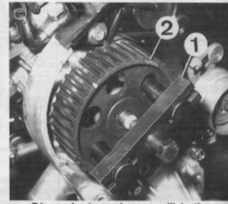
Dépose du pignon de pompe d'injection 1. Extracteur - 2. Pignon.
