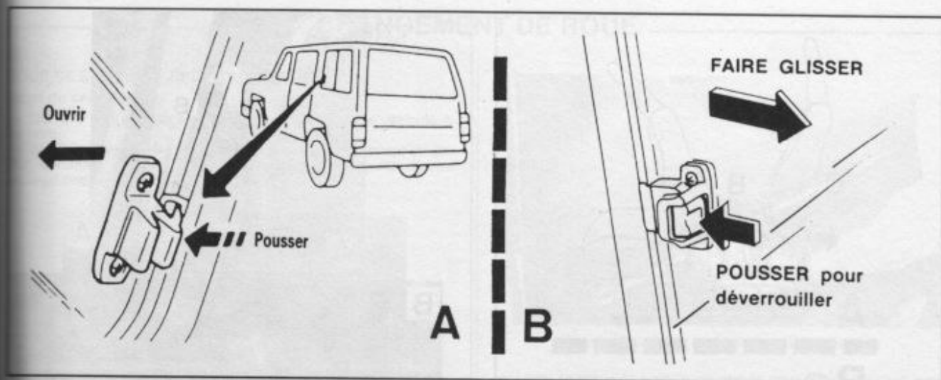
Glaces arrière coulissantes A. Sur 260 - B. Sur GR.
