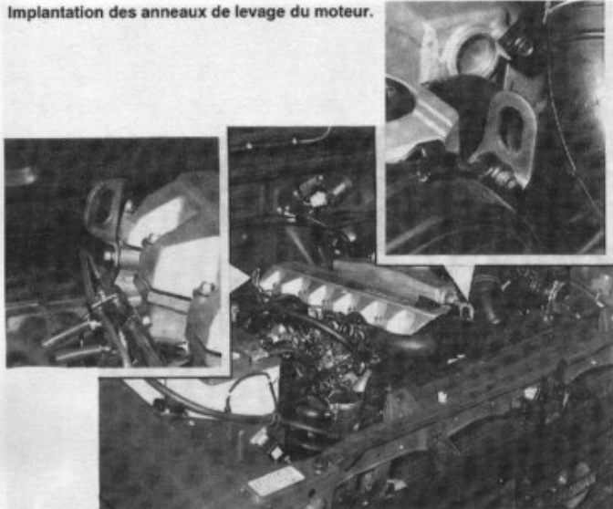
Implantation des anneaux de levage du moteur.
