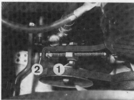
Réglage de la tension de la courroie de pompe d'assistance.
