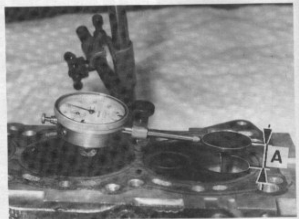
Contrôle du jeu guide-soupape A. = 15 mm.
