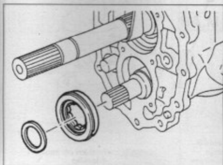
Extraction de la cuvette extérieure de roulement arrière d'arbre intermédiaire.
