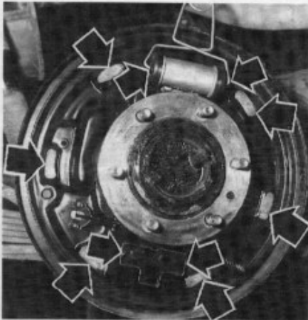
Repose des segments de frein Zones d'appui des segments à enduire de graisse.
