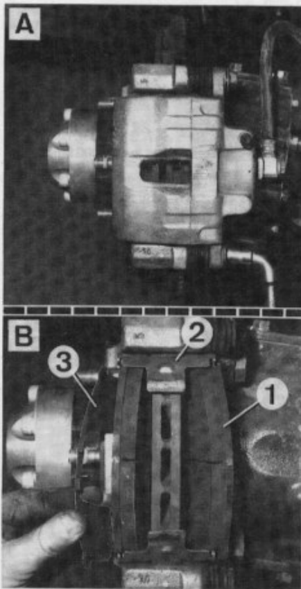
Remplacement des plaquettes de freins A. Dépose de la vis de colonnette inférieure - B. Dépose des plaquettes. 1. Plaquette - 2. Ressort de maintien - 3. Plaque anti-bruit.
