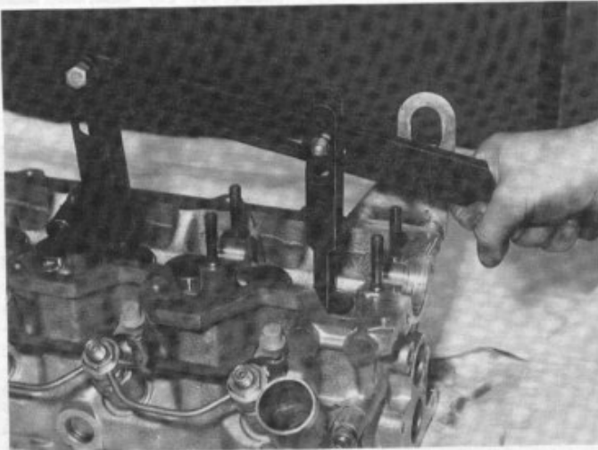
Dépose des soupapes à l'aide du compresseur.
