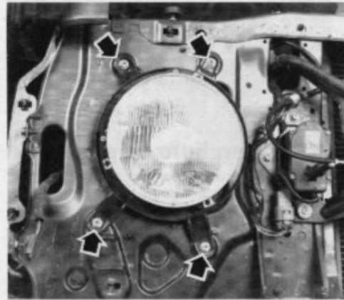
Vis de fixation d'un projecteur de Patrol 260
