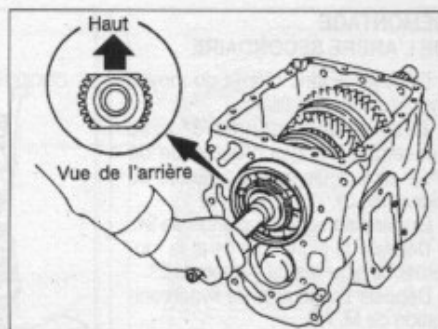
Dépose de l'arbre primaire (placer le méplat du pignon d'embrayage orienté vers le haut).
