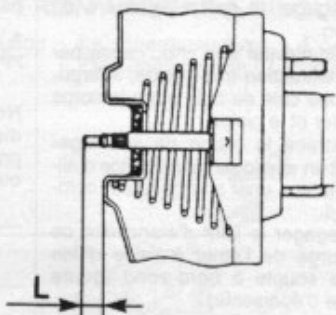
Contrôle du servofrein 1. Pompe à vide - L. Dépassement de la tige de sortie à mesurer.
