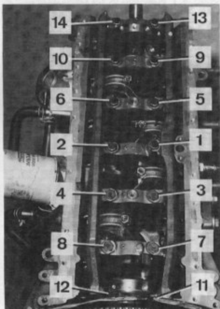
Ordre de serrage des vis de la rampe de chapeau de paliers et repérage de paliers.
