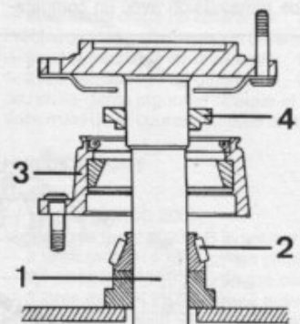
Remontage d'un arbre de roue arrière 1. Arbre - 2. Roulement - 3. Porte-roulement - 4. Entretoise.
