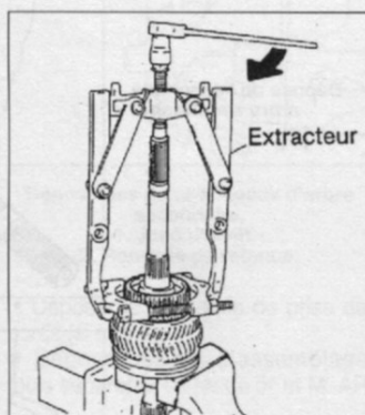
Extraction du pignon de M. AR.
