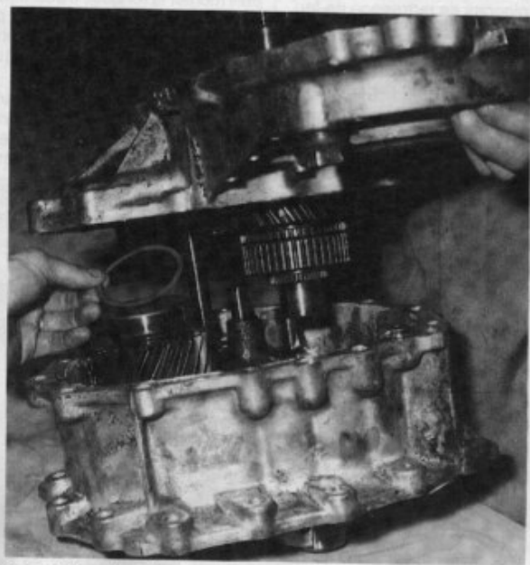
Assemblage des demi-carters de pignonerie. Ne pas oublier la rondelle de réglage de l'arbre intermédiaire.
