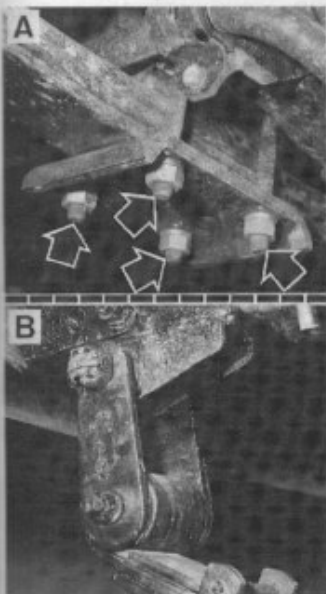
Fixations d'un ressort à lames A. Fixation sur essieu - B. Jumelle avant. Flèches : Ecrou des brides.
