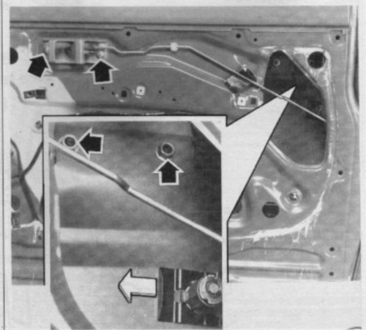
Fixation d'un système d'ouverture de porte de Patrol 260
