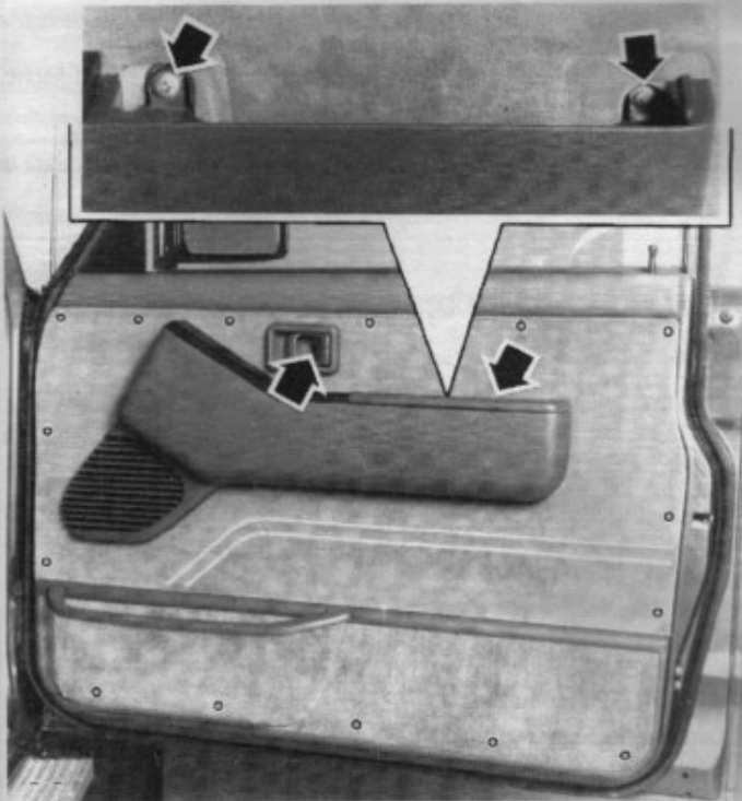
Points de fixation d'une garniture de porte (Patrol GR)
