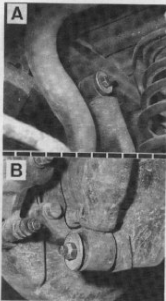
Fixations d'un amortisseur (Patrol GR) A. Supérieure - B. Inférieure.
