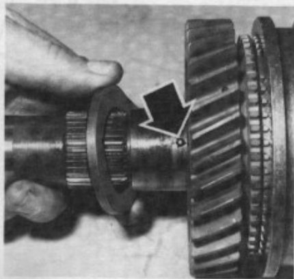
Montage de la rondelle de butée Flèche : Bille anti-rotation.
