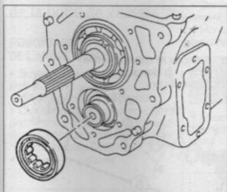
Extraction de la cuvette extérieure de roulement avant d'arbre intermédiaire.
