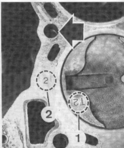
Repérage piston-cylindre Flèche : Côté pompe d'injection - 1. Repère des pistons - 2. Repères des diamètres des cylindres.
