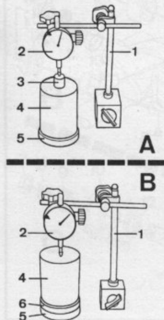
Mesure de l'épaisseur des roulements (pont C 200) 1. Support de comparateur - 2. Comparateur - 3. Cale étalon - 4. Poids - 5. Cage de roulement (opposé au côté mesuré) - 6. Roulement mesuré.
