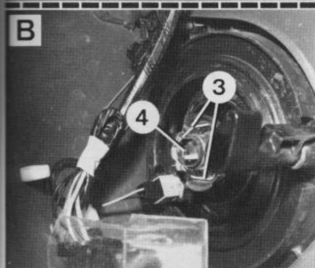
Remplacement d'une lampe de projecteur (Photo RTA) A. 1 : Connecteur - 2. Capuchon. B. 3 : Ressort de maintien - 4. Lampe.
