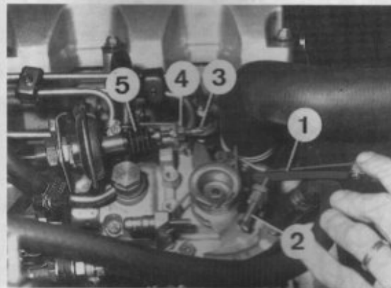
Réglage de l'amortisseur de fermeture 1. Cales - 2. Vis de réglage de régime de ralenti - 3. Vis de butée - 4. Contre-écrou - 5. Amortisseur de fermeture.
