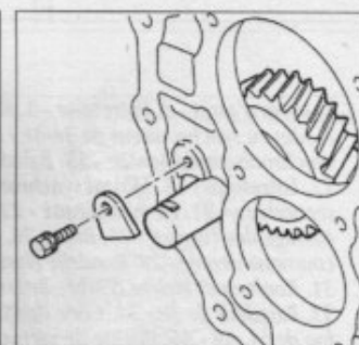
Dépose de la plaque de verrouillage de l'arbre de pignon fou de M. AR.
