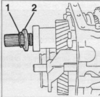
Dépose des demi-anneaux d'arbre secondaire. 1. Jonc d'arrêt - 2. Rondelle de retenue.
