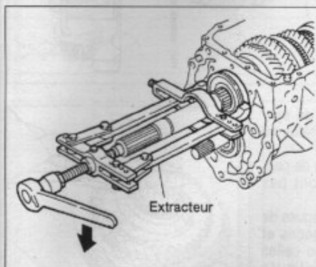
Extraction du roulement d'arbre secondaire.
