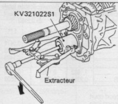
Extraction de la bague du pignon de 5 e .
