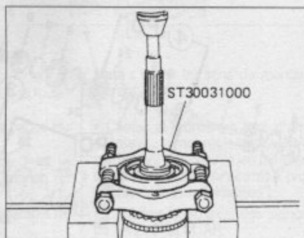
Dépose de la plaque de verrouillage de l'arbre de pignon fou de M. AR.
