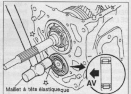
Repose de la cuvette extérieure de roulement avant d'arbre intermédiaire.
