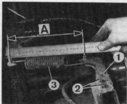
Réglage du limiteur 1. Levier - 2. Vis de réglage - 3. Ressort - A. Longueur du ressort 242 mm (Patrol 260), 221 mm (Patrol GR).
