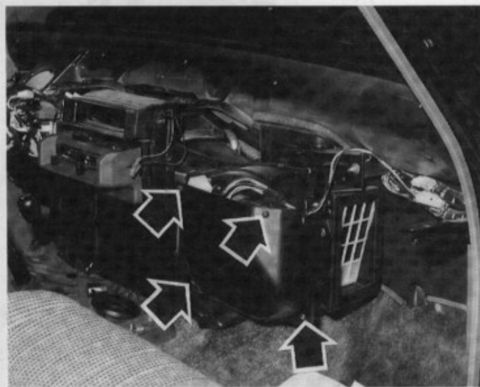
Implantation des fixations à déposer pour accéder au radiateur de chauffage.
