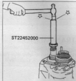
Repose de l'entretoise d'arbre secondaire et du roulement arrière d'arbre secondaire.
