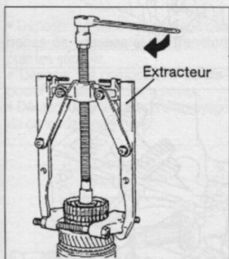
Extraction du pignon de 3 e avec l'ensemble de synchronisation de 3 e /4 e et le roulement à aiguilles du pignon de 3 e .
