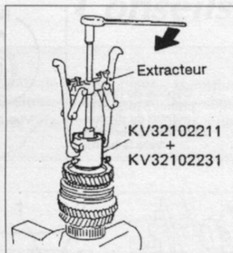
Extraction de la bague du pignon de 3 e .
