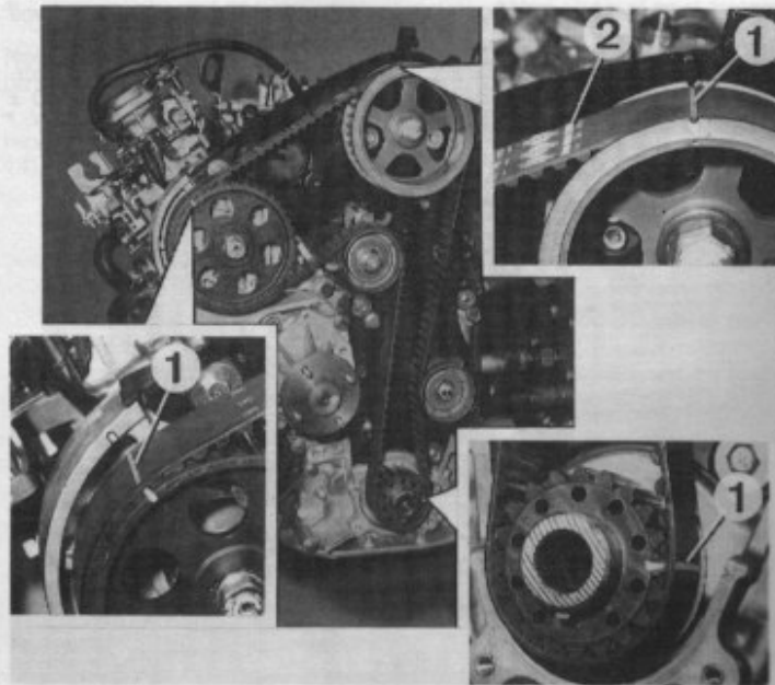
Repère de calage de la distribution 1. Repère de la courroie - 2. Flèche à diriger côté carter.
