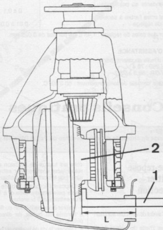
Contrôle du dispositif de blocage (pont H 233 B à blocage) 1. Règle - 2. Porte-satellites - L. Dis- tance à mesurer.
