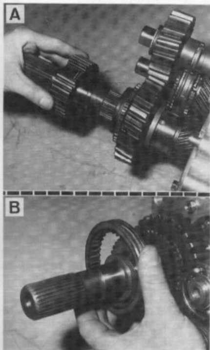
A. Sens de montage du moyeu de M.A.R - B. Sens de montage du baladeur de M.A.R.
