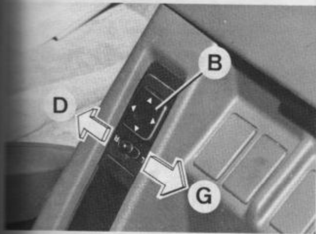
Réglage électrique des rétroviseurs extérieurs sur GR (Photo RTA) B. Sélection du rétroviseur droit - G. Sélection du rétroviseur gauche -B. Bouton de réglage de l'orientation.
