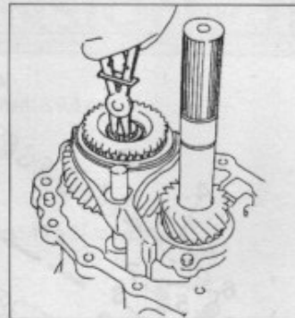
Choix d'un jonc d'arrêt pour minimiser le jeu du jonc arrière du pignon de renvoi de 5 e .
