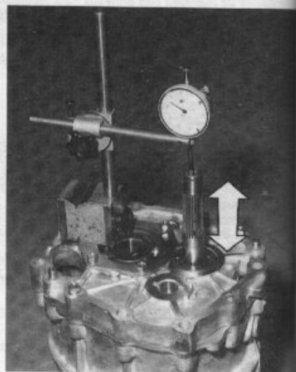
Mesure du jeu axial de l'arbre intermédiaire.
