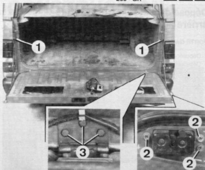
Déshabillage d'une porte arrière de Patrol 260
