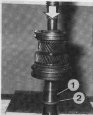
Montage de la bague intérieure du roulement à aiguilles du pignon de 1 re 1. Bague intérieure - 2. Rondelle de butée.
