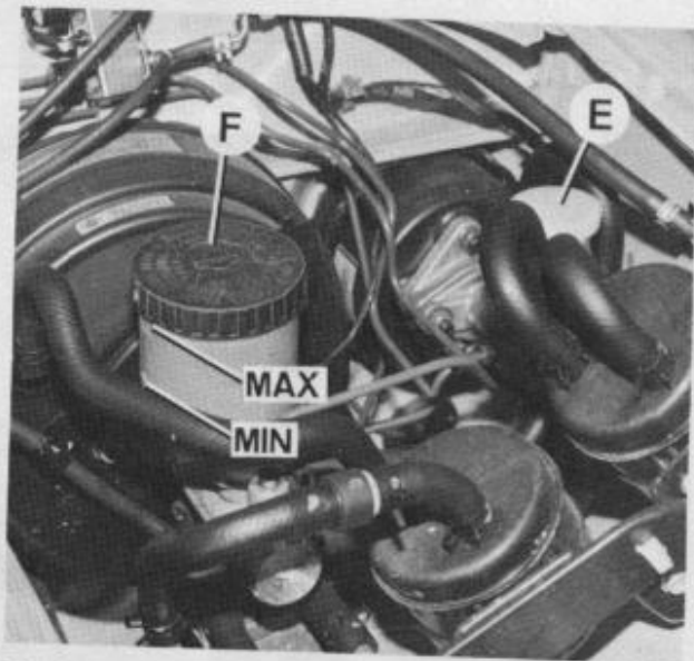
Réservoirs du liquide de frein (F) et d'embrayage (E) sur GR (Photo RTA) Emplacement identiques sur 206.
