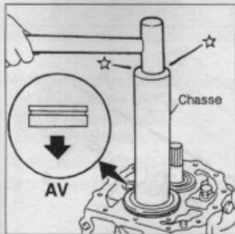
Repose du roulement d'arbre secondaire comme indiqué.
