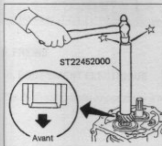
Repose du pignon de 5 e comme indiqué.
