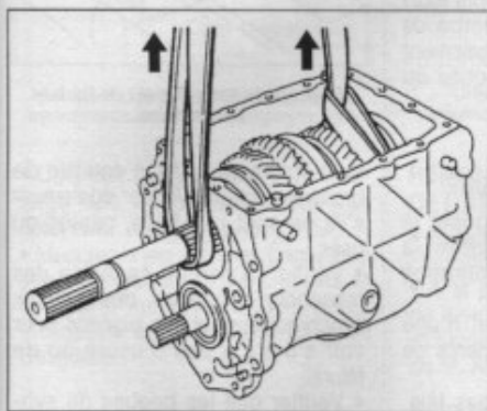
Soutien de l'arbre secondaire.
