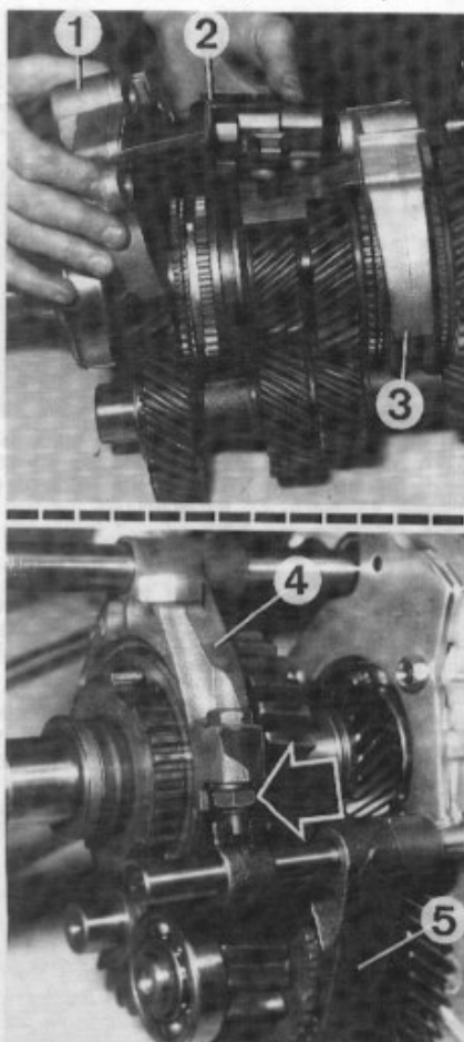
Montage des commandes de vitesses 1. Fourchette de 3 e /4 e - 2. Doigt de sélection et interdiction - 3. Fourchette de 1 re /2 e - 4. Fourchette de M.A.R - 5. Fourchette de 5 e .
