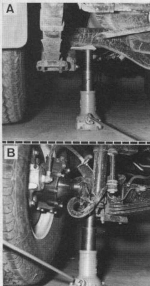
Mise en place du cric (Photos RTA) A. A l'arrière - B. A l'avant.
