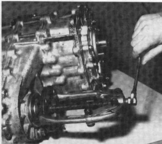
Extraction d'une bride de sortie.
