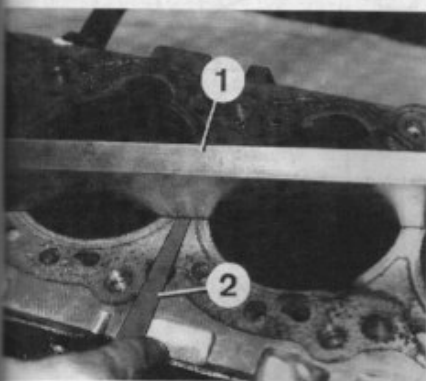
Contrôle de la planéité de la culasse 1. Règle - 2. Jauge d'épaisseur.
