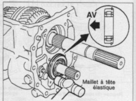
Repose de la cuvette extérieure de roulement arrière d'arbre intermédiaire.
