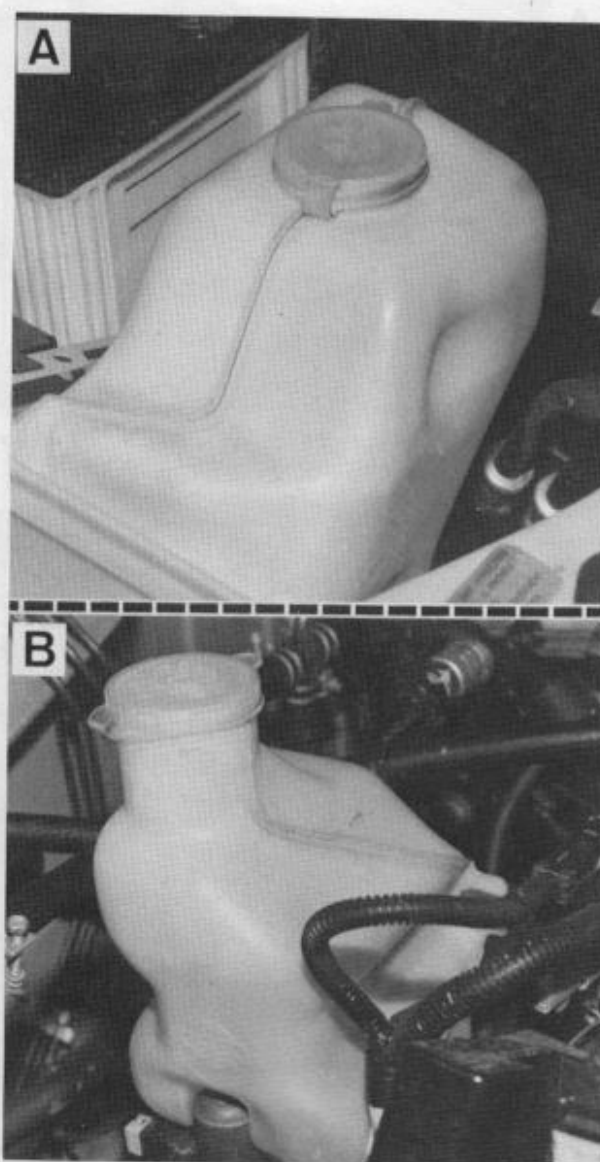
Réservoirs de lave-glaces sur GR (Photo RTA) A. Pare-brise - B. Phares.
