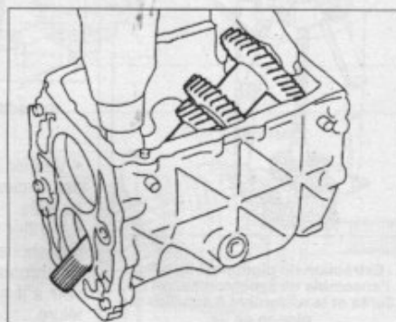
Dépose de l'ensemble arbre intermédiaire.
