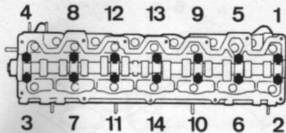
Repérage des paliers d'arbre à cames et ordre de desserrage.
