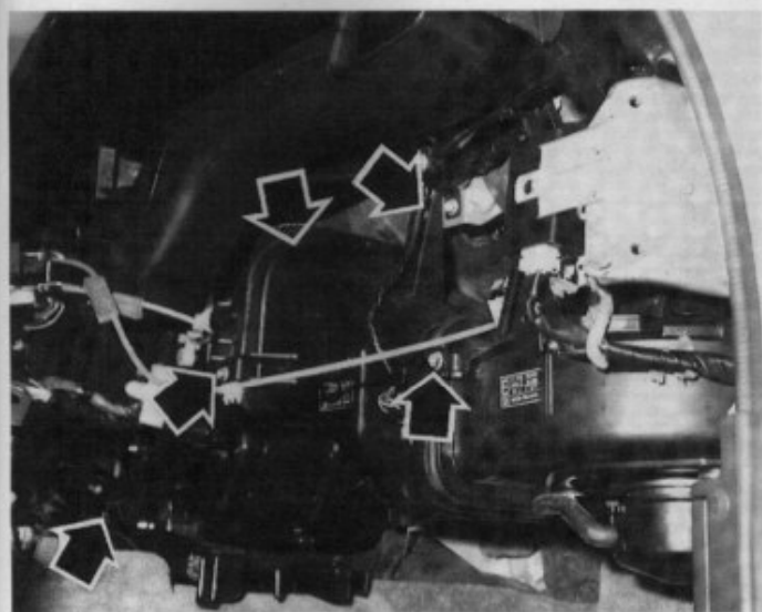
Vis de fixation du carter de bloc chauffage (Patrol 260).
