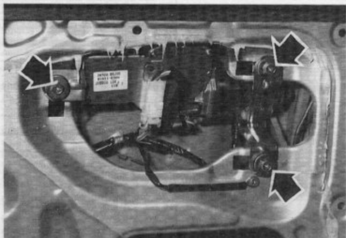
Vis de fixation du mécanisme d'essuie-glace arrière (Patrol GR).
