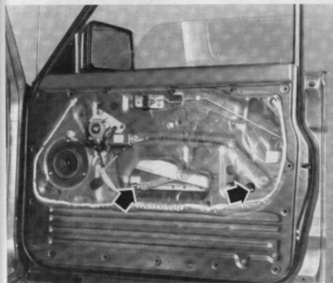
Vis de fixation de la vitre sur le mécanisme de lève-vitre (Patrol GR)
