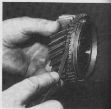
Contrôle de l'usure d'une bague de synchro.
