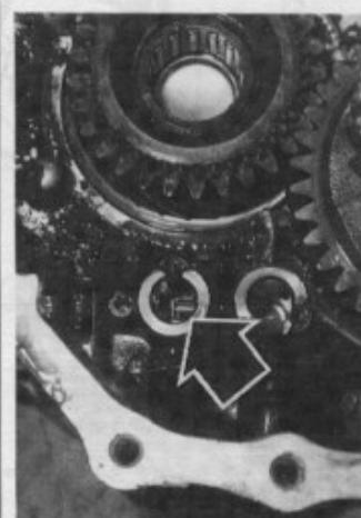
Montage du bonhomme d'interdiction.
