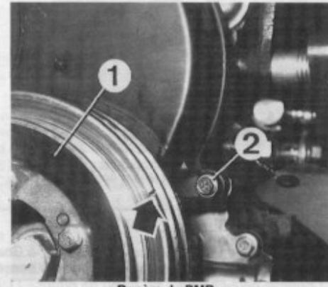
Repère de PMB 1. Poulie de vilebrequin - 2. Vis.
