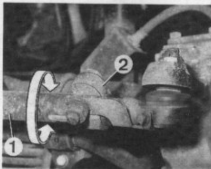
Réglage du parallélisme 1. Barre d'accouplement - 2. Collier de fixation.
