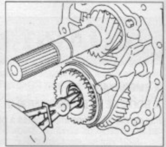
Extraction du jonc d'arrêt arrière du pignon de renvoi de 5 e .
