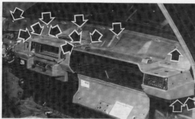
Vis de fixation du châssis de planche de bord (Patrol 260).
