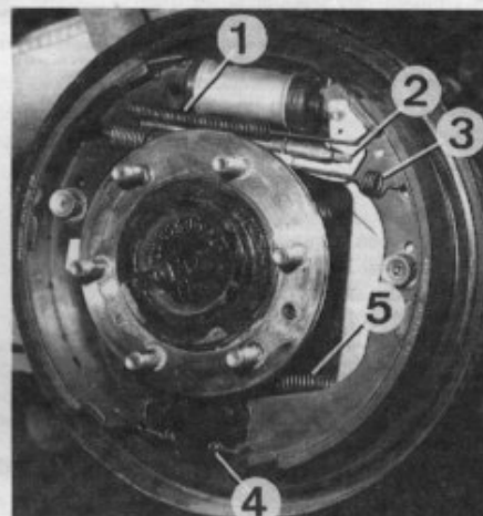
Dépose des segments de frein
