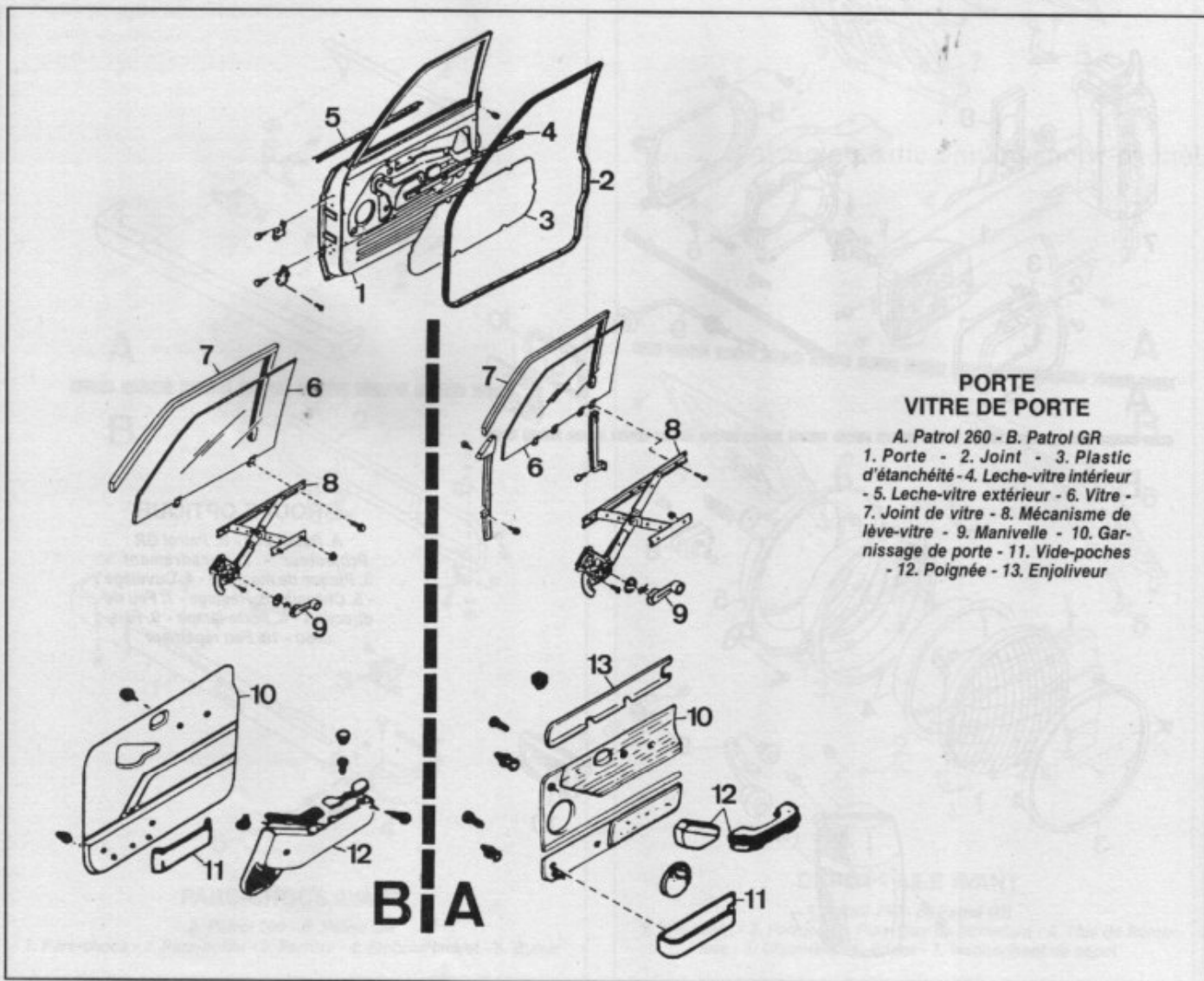
Points de fixation d'une garniture de porte (Patrol 260)
