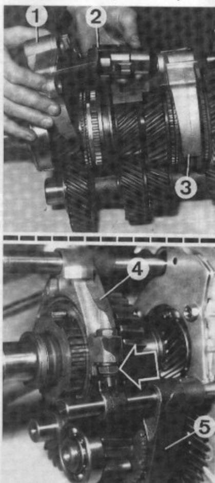
Montage des commandes de vitesses 1. Fourchette de 3 3/4 - 2. Doigt de sélection et interdiction - 3. Fourchette de 1 1/2 - 4. Fourchette de M.AR - 5. Fourchette de 5 e .
