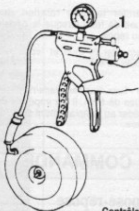
Contrôle du servofrein 1. Pompe à vide - L. Dépassement de la tige de sortie à mesurer.
