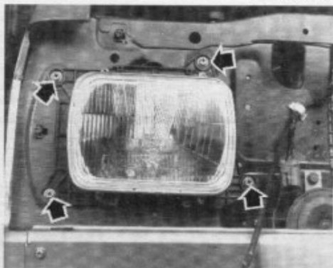
Vis de fixation d'un projecteur de Patrol 260
