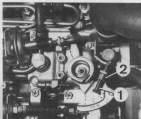
Réglage du régime de ralenti 1. Vis de réglage - 2. Contre-écrou.
