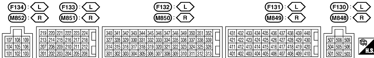
ECM (moteur TD27Ti)
