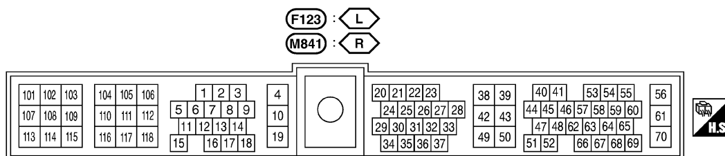
ECM (moteur ZD30DDT)
