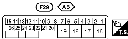
ACTIONNEUR ET DISPOSITIF ELECTRIQUE ABS (BOITIER DE COMMANDE)
