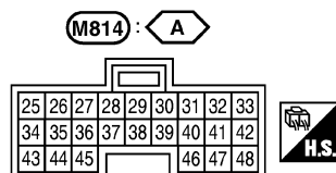
TCM (boîtier de commande de transmission)
